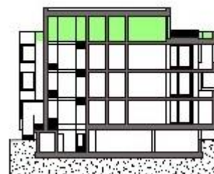
ŘEZ OBJEKTEM
