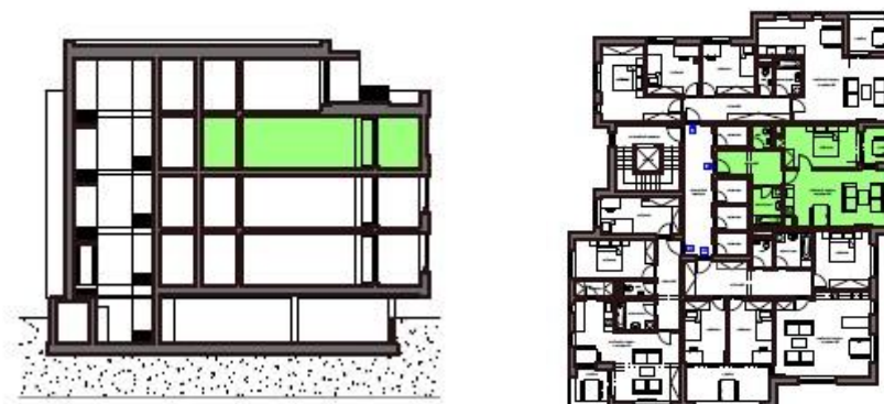
ŘEZ OBJEKTEM
